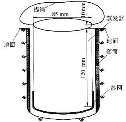
图 1 蒸发器结构及安装示意
