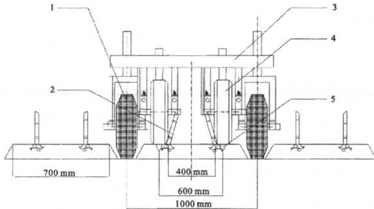
1. 稳定装置 Stabilization device; 2. 直立根茬 Stand-up stubble; 3. 机架 Framework; 4. 镇压轮 Press wheel; 5. 开沟器 Opener
