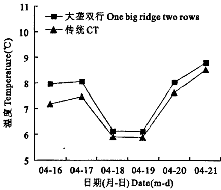
图 3 10 cm 处两种播种模式的地温对比
