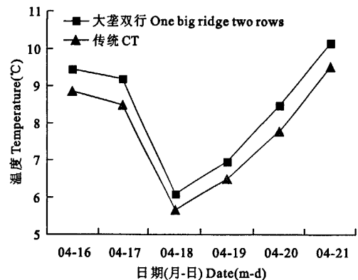
图 2 5 cm 处两种播种模式的地温对比
