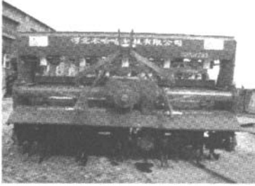
图4 2BMFS-5/10型小麦免耕播种机 Fig.4 2BMFS-5/10 wheat no-till seeder
