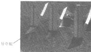
图3 玉米免耕播种机导草棍
