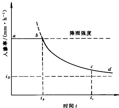
图 1 稳定降雨强度下的入渗过程
