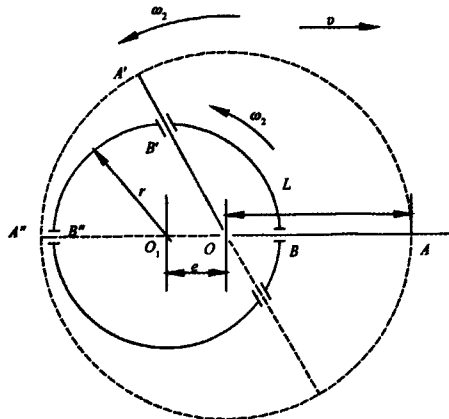
图 2 伸缩式拨杆运动分析示意图
