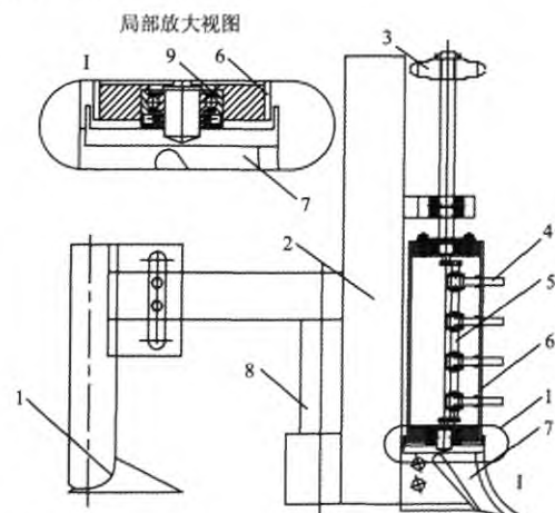
1. 播种开沟器 2. 铲柄 3. 链轮 4. 拨杆 5. 偏心轴 6. 转筒 7. 开沟器 8. 施肥管 9. 轴承
